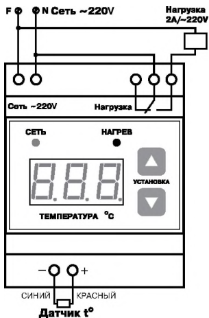
Рис.2 Схема подключения терморегулятора
