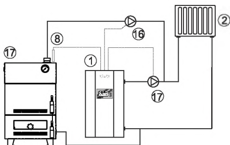
Рис.6 Упрощенная схема подключения котла в режиме вспомогательного.
