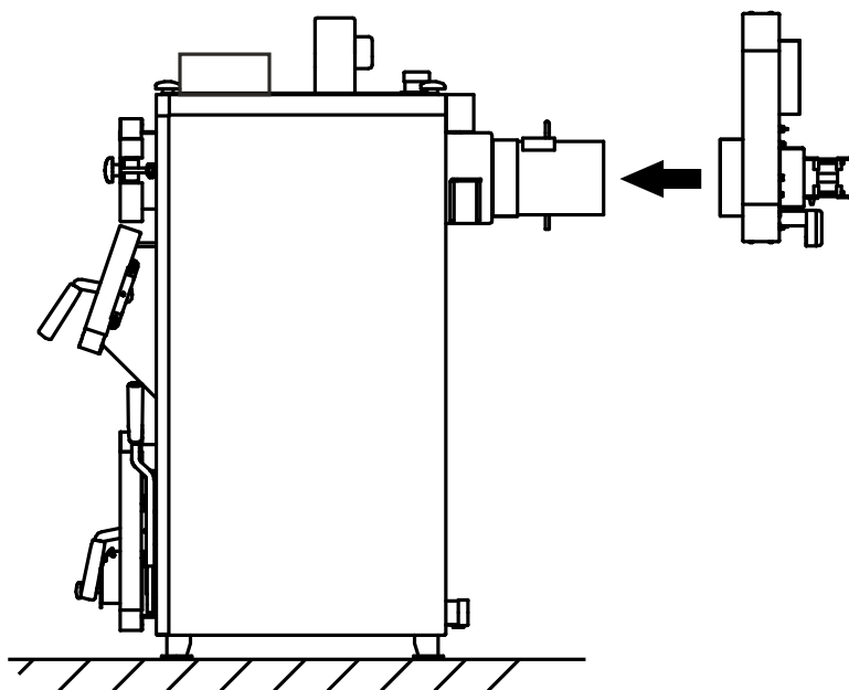
Рис.3. Вариант установки дымососа
