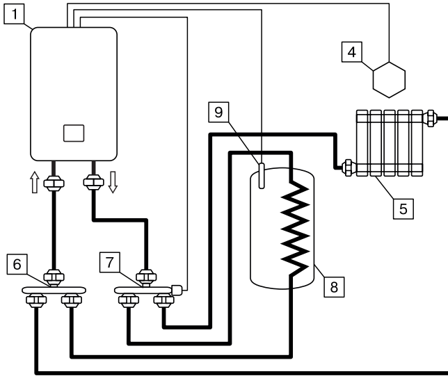
Рис.6 Упрощённая схема подключения миникотельной в режиме «Отопление-ГВС».
